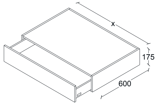
GABINETE CHICO. 1 CAJON (H173). H175, F600.
