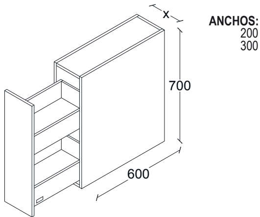
GABINETE BOTELLERO. 2 CORREDERAS. H700, F600.
