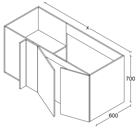
GABINETE RINCONERO RECTO FREGADERO IZQUIERDO. 2 PUERTAS. H700, F600.
