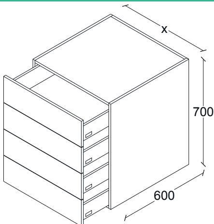
GABINETE 4 CAJONES (H175). H700, F600.
