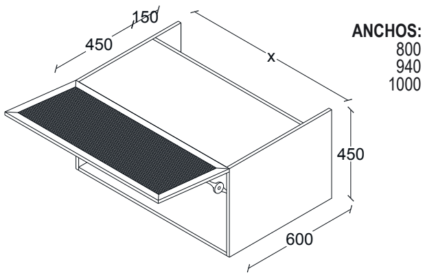
ALACENA SOBRE REFRIGERADOR HORIZONTAL. SIN ENTREPAÑO H450, F600.
