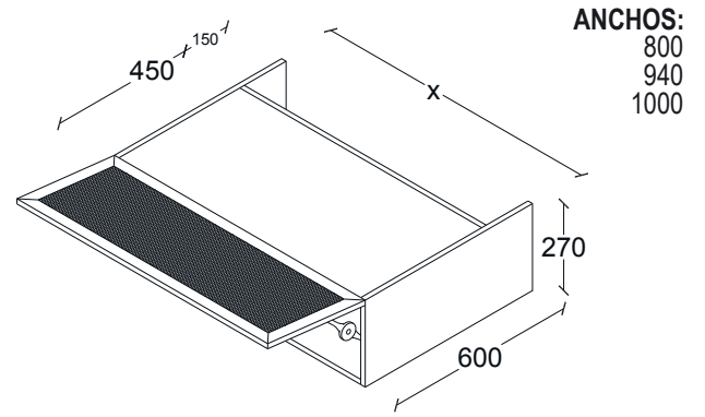
ALACENA SOBRE REFRIGERADOR HORIZONTAL. SIN ENTREPAÑO. H270, F600.
