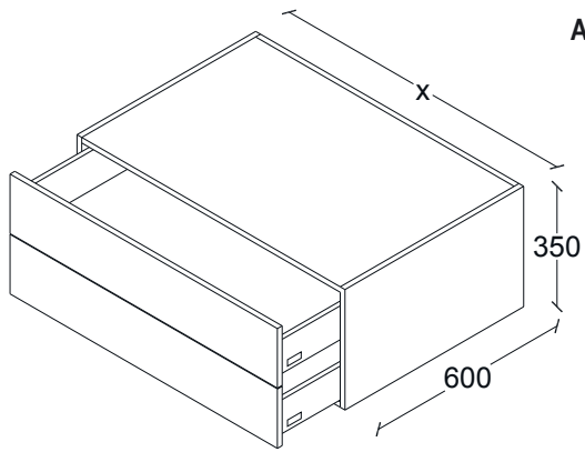
GABINETE CHICO. 2 CAJONES (H173). H350, F600.
