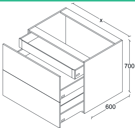
GABINETE DINAMICO. 1 CAJÓN (H350), 1 CAJÓN (H175) Y 1 CAJÓN INTERIOR. H700, F600.
