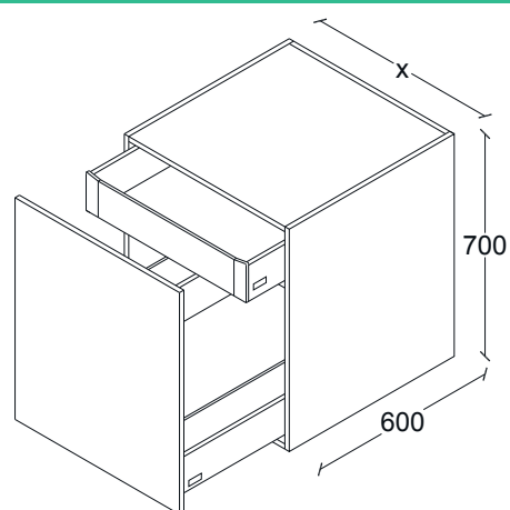
GABINETE BASURERO. 1 CAJON (FRENTE 698) Y 1 CAJÓN INTERNO. H700, F600.
